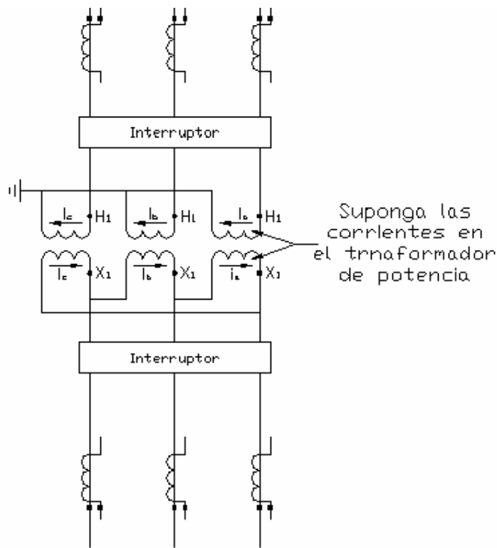
Fig. 1. Desarrollo de las conexiones de los TC para protección diferencial del transformador, primer paso.
