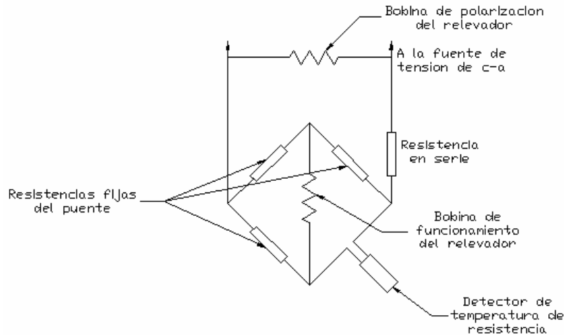
Fig. 17. Protección de sobrecalentamiento del estator con detectores de temperatura de resistencia.
