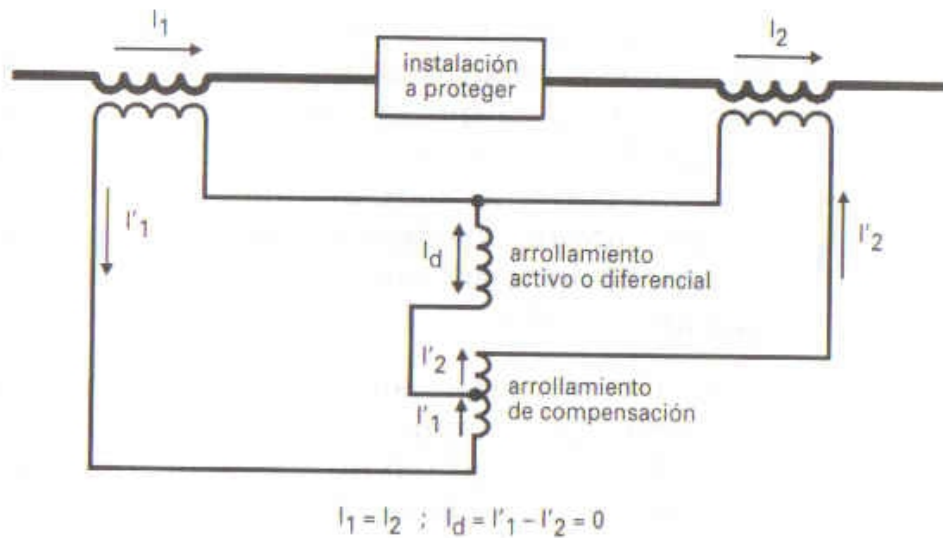
Actuación de la protección diferencial compensada en caso de falla con alimentación por un extremo
