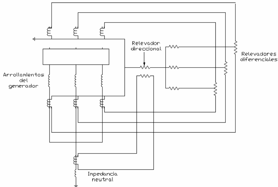
Fig. 13. Protección sensible contra fallas a tierra en el estator para generadores.
