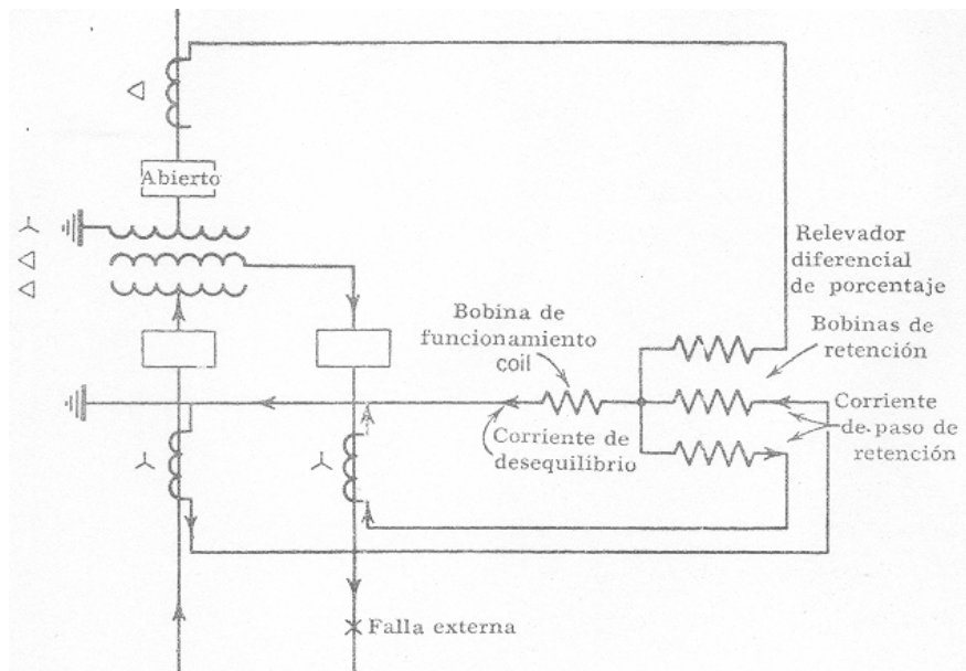
Fig. 9Ejemplo de la ventaja de un relevador para tres arrollamientos con un transformador de tres
