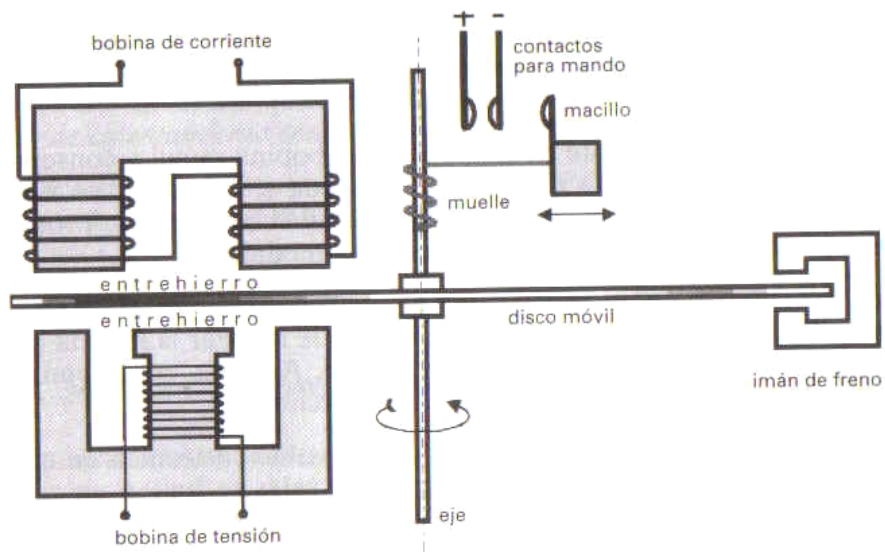
Esquema constructivo de un relé de protección de inducción
