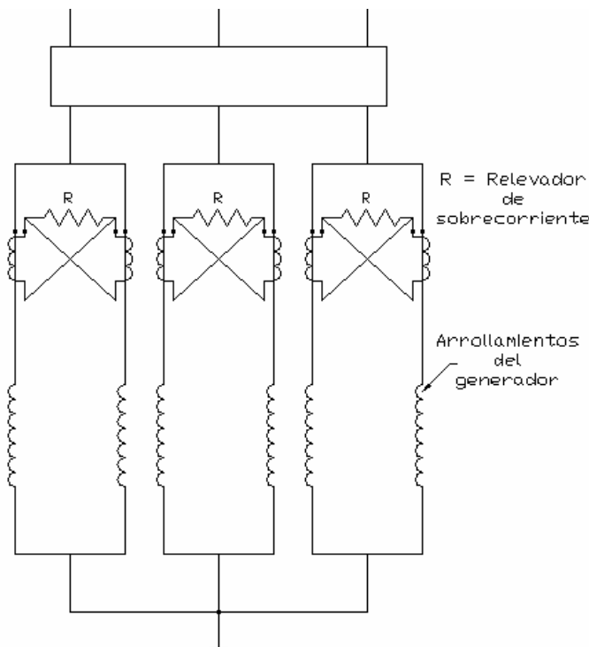
Fig. 9. Protección de fase auxiliar para un generador multicircuito.
