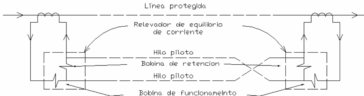
Fig. 5 Dibujo esquemático del principio de la tensión de oposición de protección por hilo piloto de c-a
