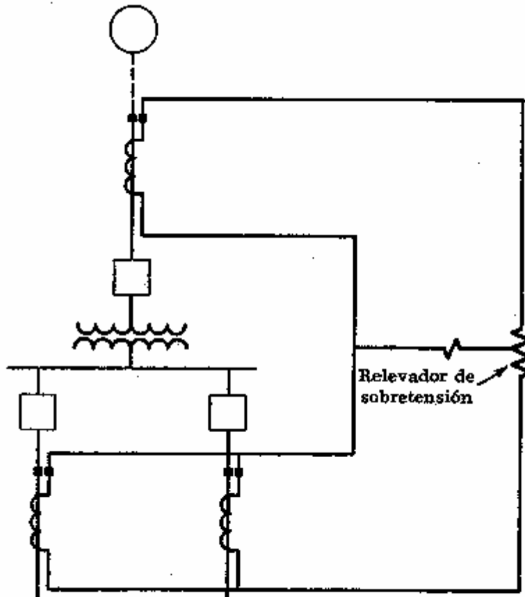
Fig. 9 Protección combinada de transformador y barra colectora con un relevador diferencial de porcentaje de dos arrollamientos.
