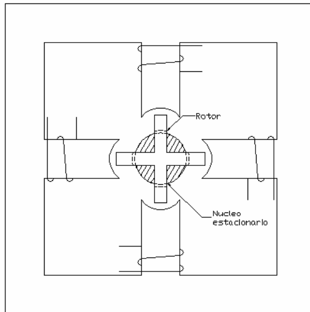
Fig. 12. Estructura de anillo doble de inducción
