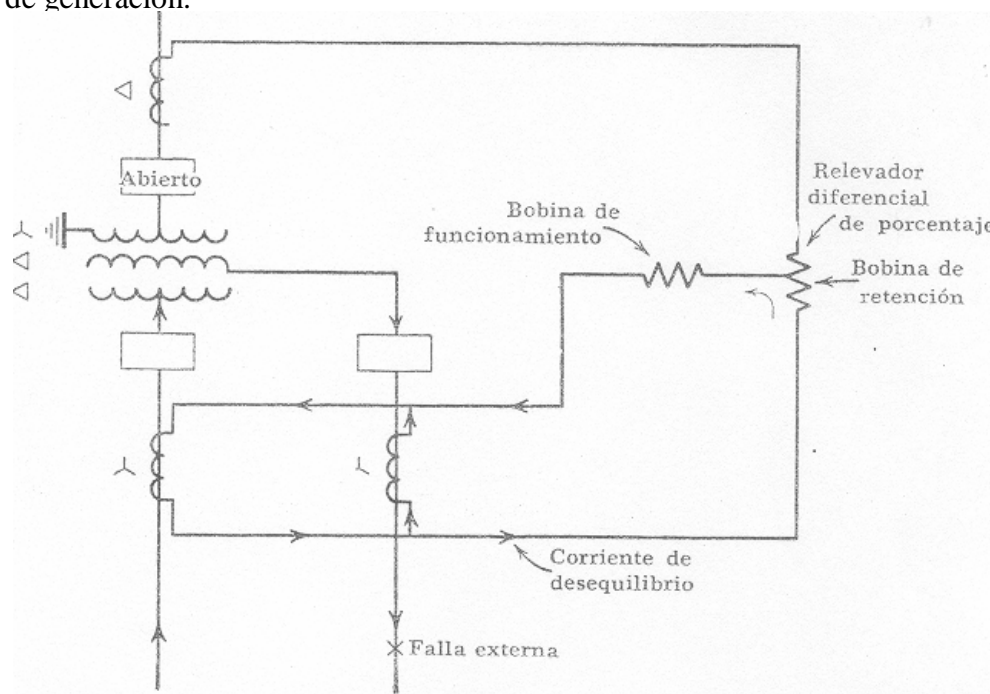
Fig. 8 Una mala aplicación de un relevador diferencial para transformador de dos arrollamientos.
