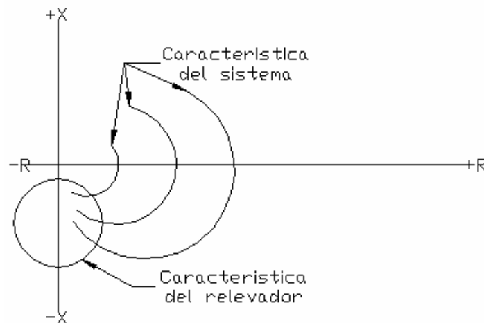
Fig. 20. Característica del relevador de pérdida de excitación y del sistema.
