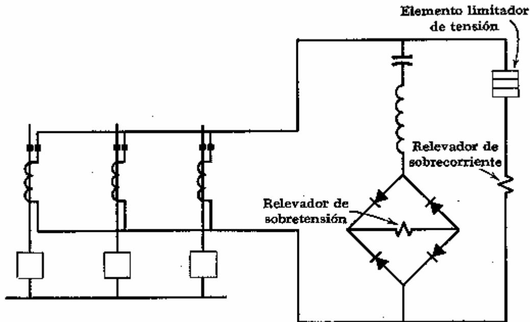
Fig. 8 Protección de barra colectora utilizando protección diferencial de corriente con relevadores de sobretensión.
