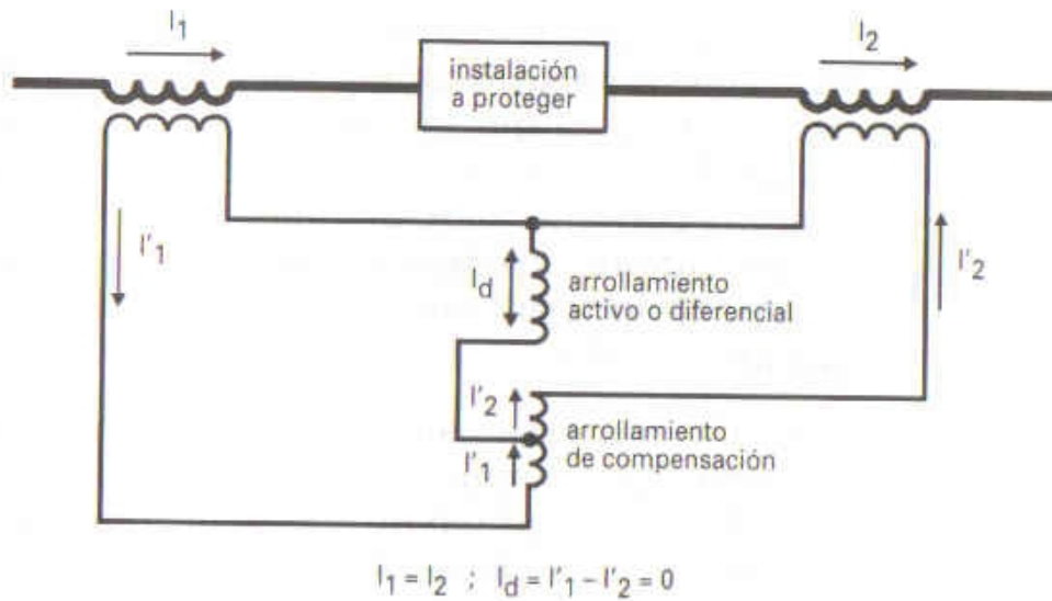
Principio de funcionamiento de la protección diferencial compensada
