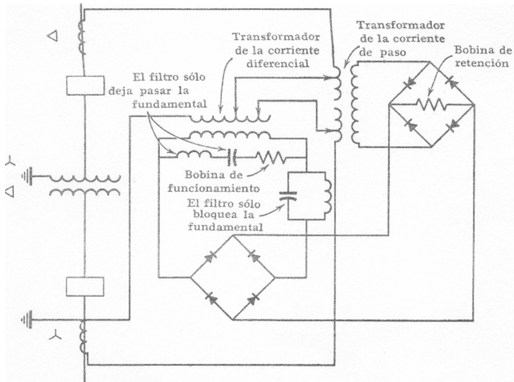
Fig. 11 Relevador diferencial de porcentaje de retención de corriente armónica
