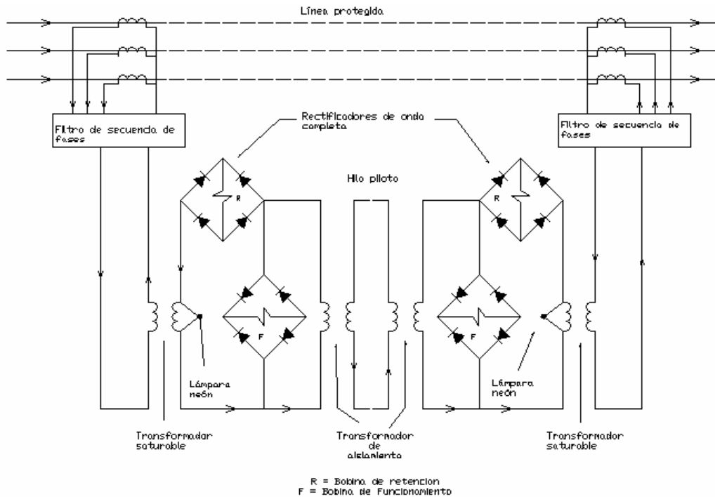
Fig. 6 Conexiones esquemáticas de un equipo de protección por hilo piloto de c-a de corriente circulante
