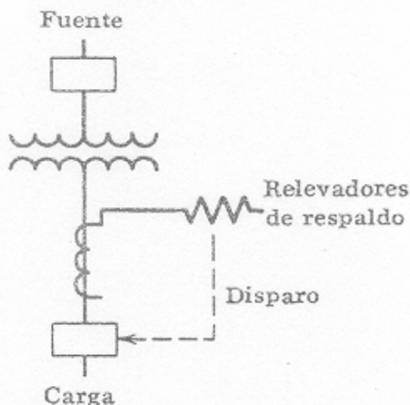
Fig. 14 Protección de respaldo para el transformador conectado a una fuente.
