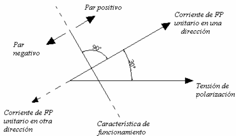
Característica típica de funcionamiento de un relevador de potencia
