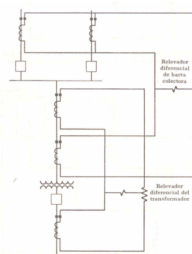
Fig. 11 Alternativa de la Fl. 10 preferida cuando las líneas de alta tensión son de estaciones diferentes.
