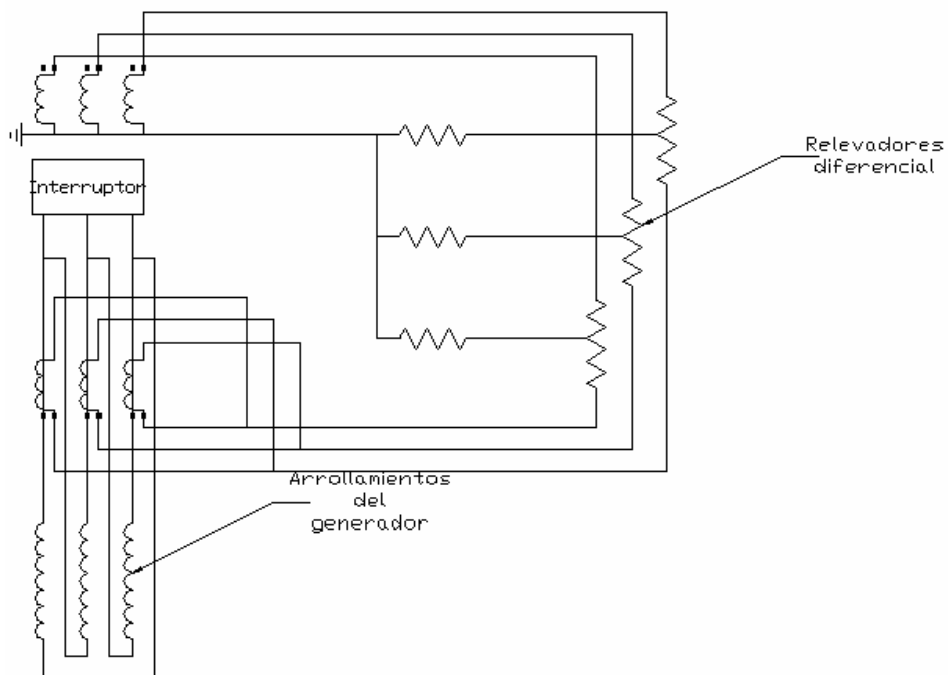
Fig. 2. Protección diferencial de porcentaje para un generador conectado en delta.
