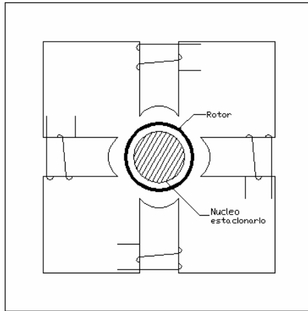
Fig. 11. Estructura de tambor de Inducción
