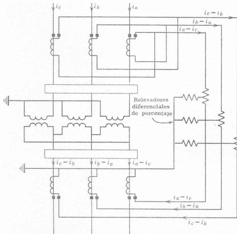
Fig. 3 Conexiones completas de la protección diferencial de porcentaje para un transformador de dos arrollamientos.
