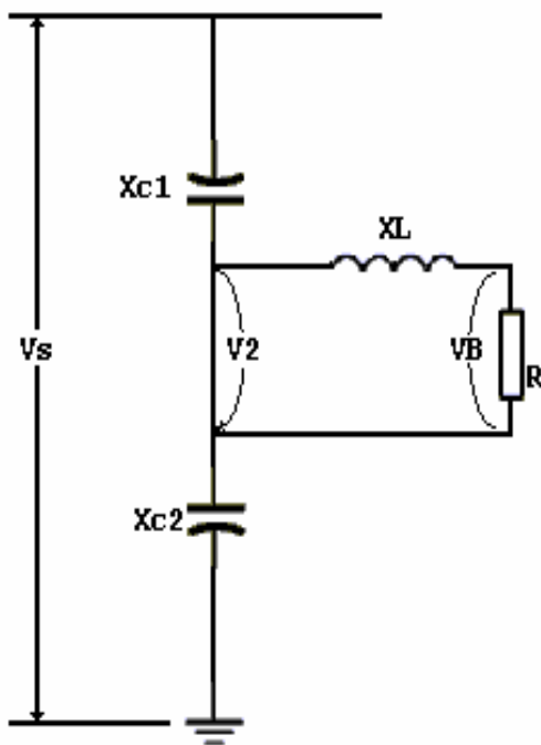
Circuito equivalente de un dispositivo de potencial clase A
