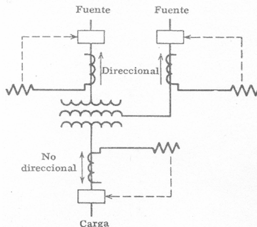
Fig. 15 Protección de respaldo con dos fuentes.
