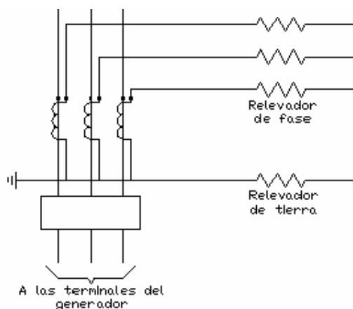
Fig. 16. Protección de sobrecorriente del estator del generador.
