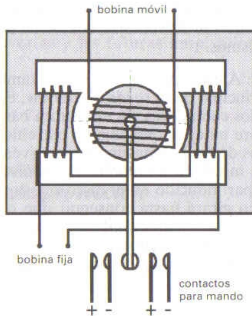
Esquema constructivo de un relé de protección electrodinámico
