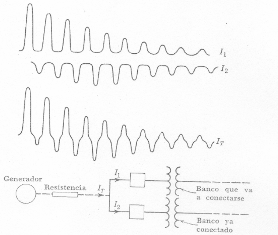
Fig. 13 Corrientes transitorias de conexión prolongadas con transformadores en paralelo.
