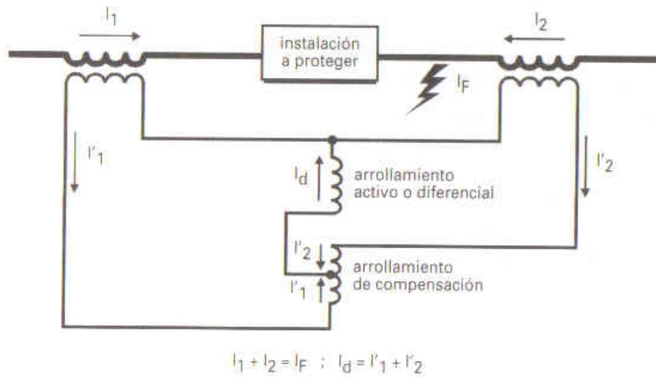
Actuación de la protección diferencial compensada en caso de falla con alimentación por los dos extremos.
