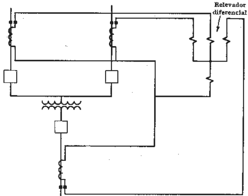
Fig. 10 Protección combinada de transformador y barra colectora con un relevador diferencial de porcentaje de tres arrollamientos.
