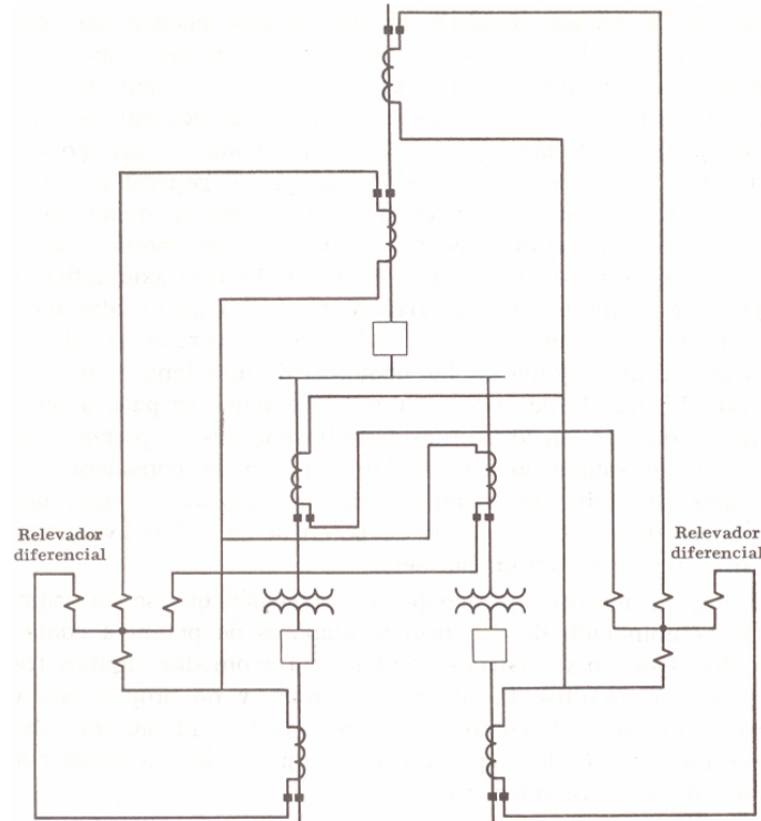
Fig. 12 Protección completa de dos transformadores y de una barra colectora con dos relevadores diferenciales de porcentaje de tres arrollamientos.
