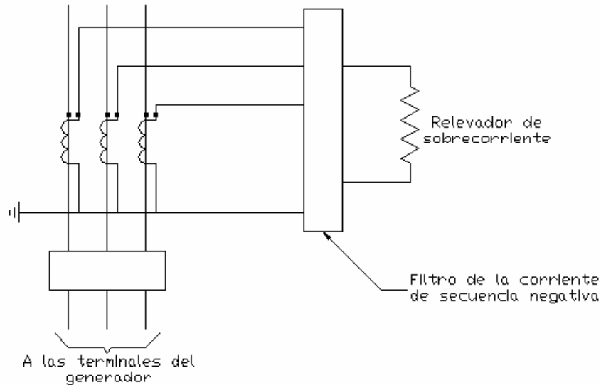
Fig. 19. Protección de sobrecorriente del estator del generador.
