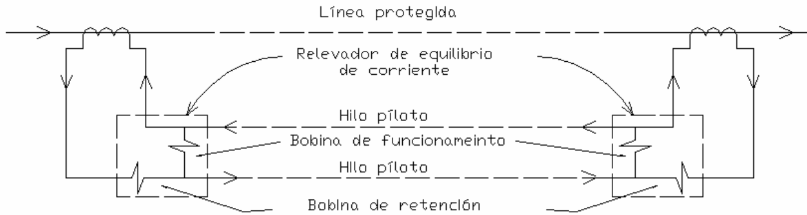
Fig. 4 Dibujo esquemático del principio de la corriente circulante de la protección por hilo piloto de c-a
