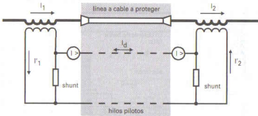
Protección diferencial longitudinal aplicada a una línea, utilizando dos relés diferenciales de sobreintensidad e hilos piloto
