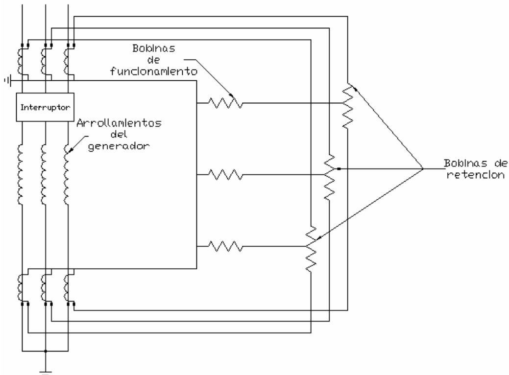
Fig. 1. Protección diferencial de porcentaje para un generador conectado en estrella.
