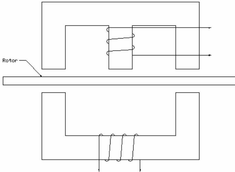
Fig. 10. Estructura de wathhorímetro
