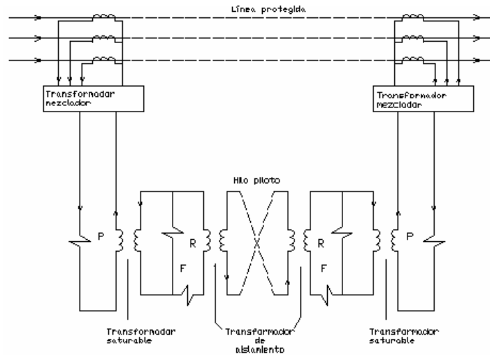
Fig. 7 Conexiones esquemáticas de un equipo de protección por hilo piloto de c-a de tensión de oposición. P = Bobina de corriente de polarización; R = Bobina de tensión de retención; F = Bobina de corriente de régimen o de funcionamiento.
