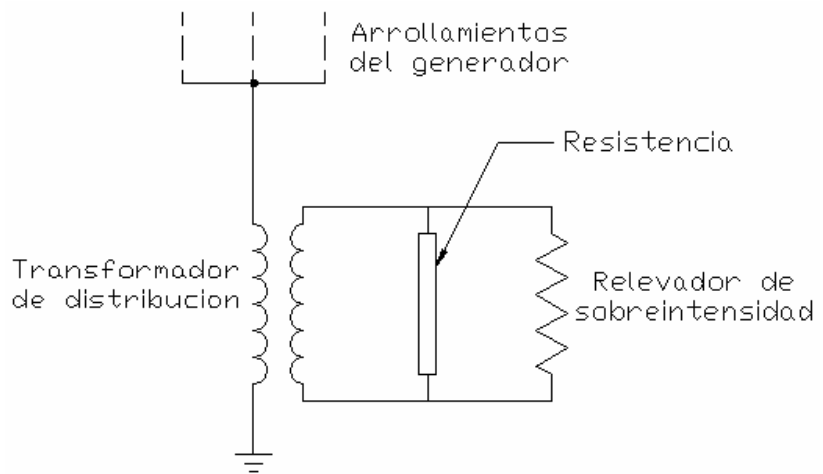
Fig. 14. protección contra fallas a tierra en el estator para unidades generadoras.
