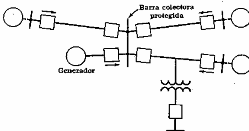
Fig. 1 Protección de barra colectora por medio de relevadores de respaldo.
