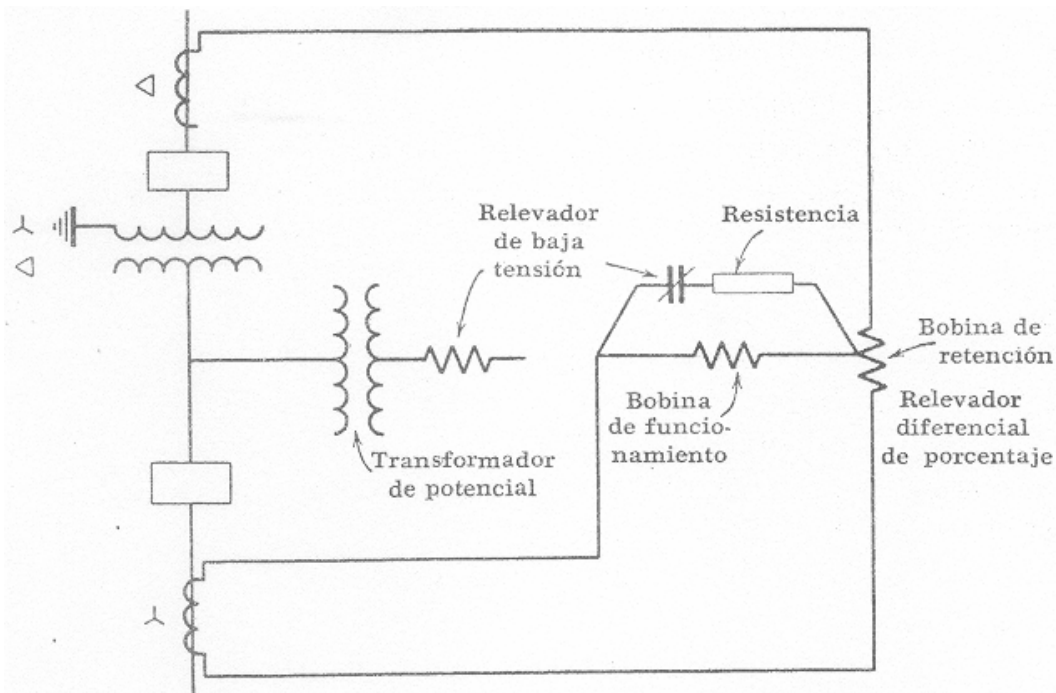
Fig. 10 Equipo de desensibilización para impedir el disparo del relevador diferencial en la corriente magnetizante transitoria de conexión
