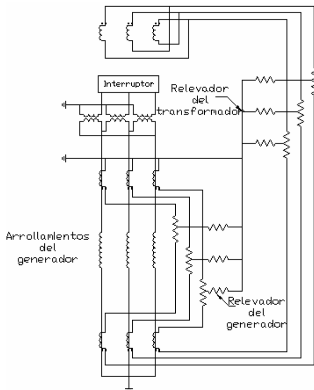
Fig. 4. Protección diferencial de porcentaje para una unidad generador-transformador. Nota: La secuencia de fases es a-b-c.
