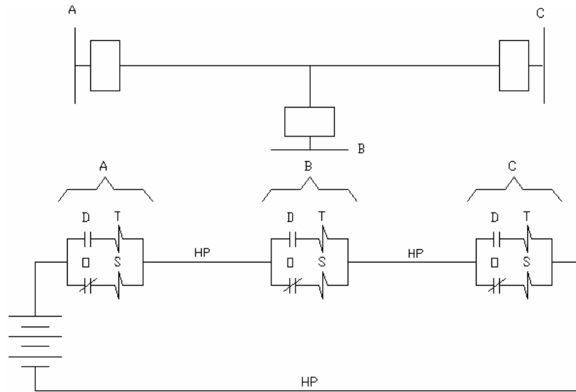
Fig. 2 Dibujo esquemático de un equipo de protección por piloto de c-d. D = relevador direccional (nho) de tensión de retención; □ = relevador de sobrecorriente; T = relevador auxiliar de disparo; S = relevador auxiliar supervisor; HP = hilo piloto.
