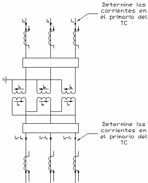
Fig. 2. Desarrollo de las conexiones de los TC para proteccion diferencial del transformador, segundo paso.
