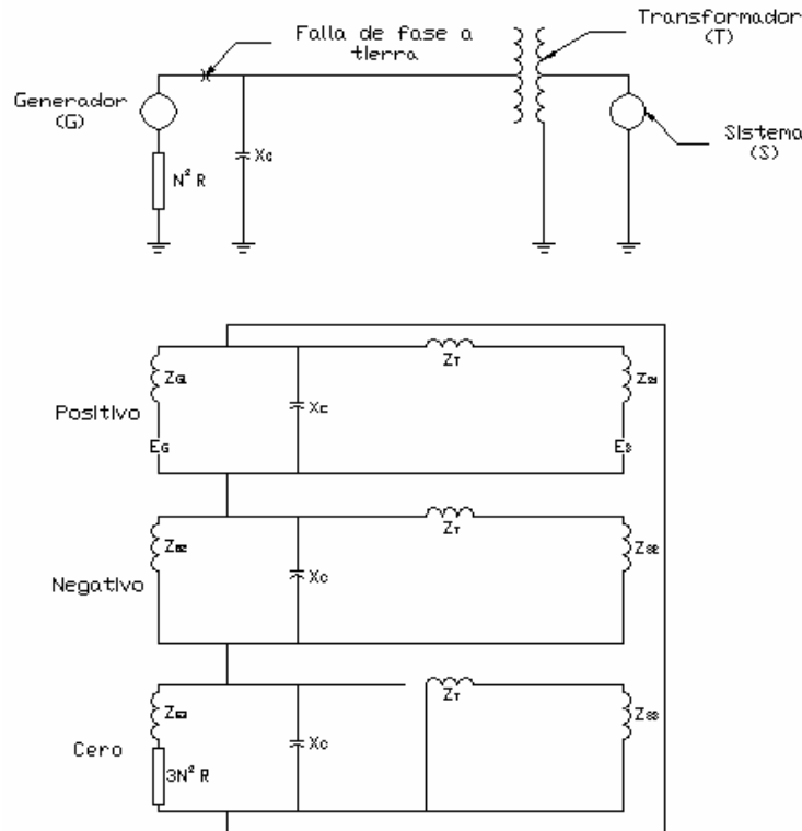
Fig. 15. (a) Diagrama unifilar de un sistema con una unidad generadora y una falla a tierra. (b) Diagrama de secuencia de fases para (a)
