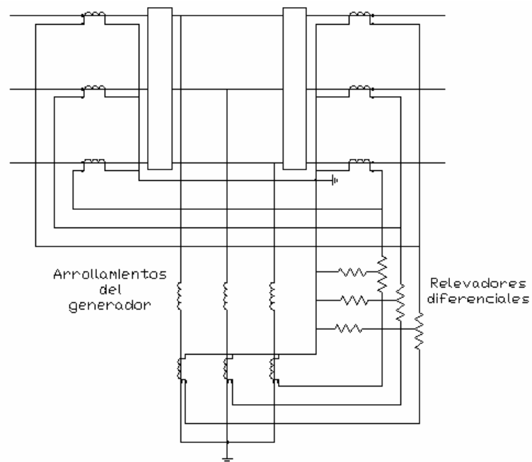
Fig. 5. Protección diferencial de generador con unas barras colectoras de doble Interruptor.
