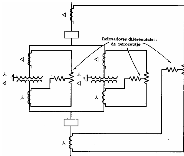
Fig. 12 La protección de bancos en paralelo con interruptores comunes.
