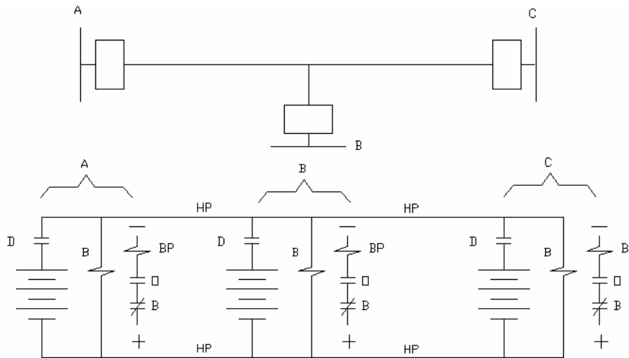
Fig. 3 Dibujo esquemático de un equipo de protección por piloto de c-d, donde la información se trasmite por el piloto. D = relevador direccional (mho) de tensión de retención; B = relevador auxiliar de bloqueo; BP = relevador de sobrecorriente; B = bobina de disparo; HP = hilo piloto.
