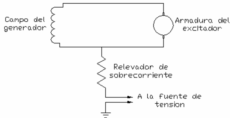
Fig. 18. Protección contra fallas a tierra en el campo del generador
