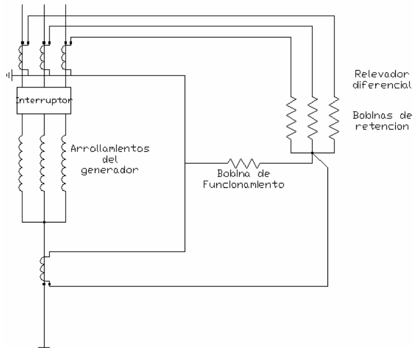
Fig. 3. Protección diferencial de porcentaje para un generador conectado en estrella con solo cuatro terminales sacadas al exterior.
