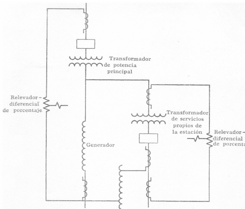
Fig. 4 Conexiones esquemáticas para la protección diferencial de los transformadores principal y de servicios propios
