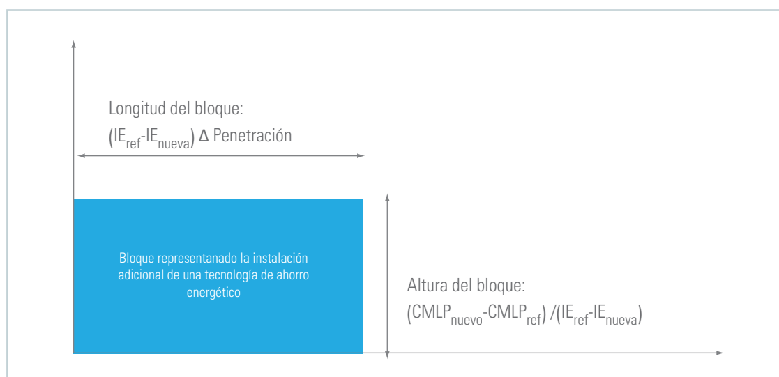
Figura 4. Altura y anchura de bloques de la curva de ahorro energético
